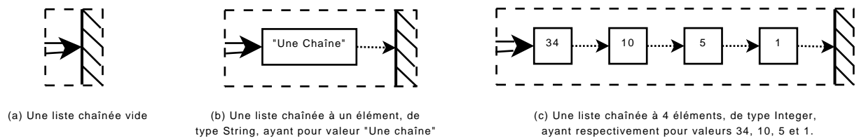
FIG. 2: Illustration de la définition d'une liste chaînée faisant apparaître le concept de maillon. Un rectangle en traits correspond à un objet dont la classe est «ListeChaînée». Un rectangle en traits pleins correspond à un objet dont la classe est «Maillon».
