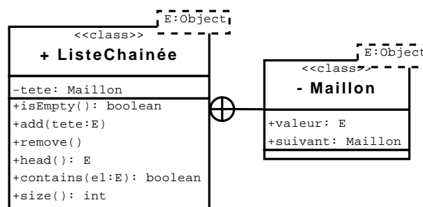
FIG. 3: Diagramme UML de la solution à la première partie du TD.
